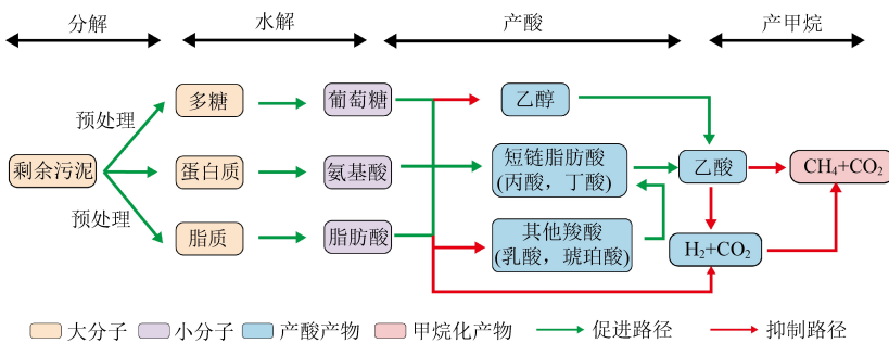
图 5 剩余污泥厌氧发酵机理图
