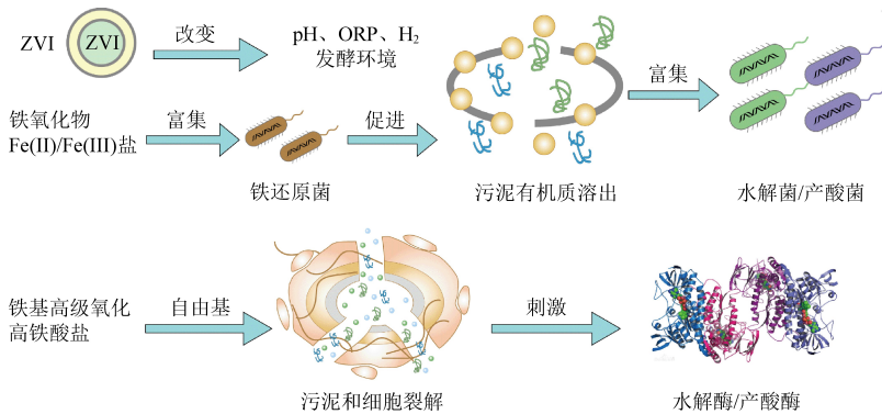
图 2 铁/铁基高级氧化促进污泥厌氧发酵示意图
