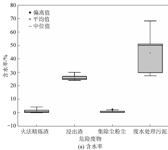
图 2 有色冶炼典型危险废物的含水率和 pH
