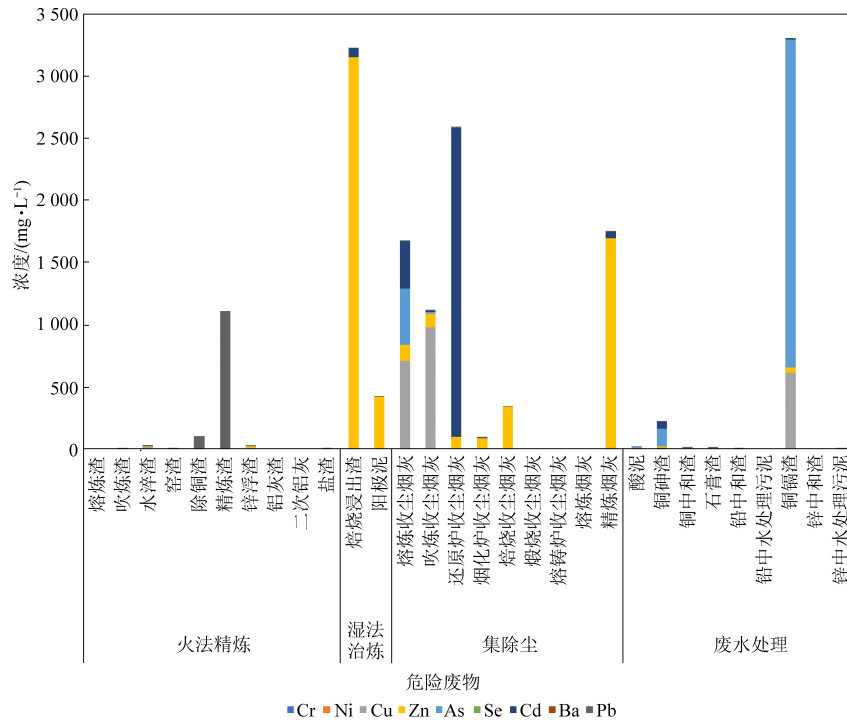
图4 有色冶炼典型危险废物的浸出浓度
