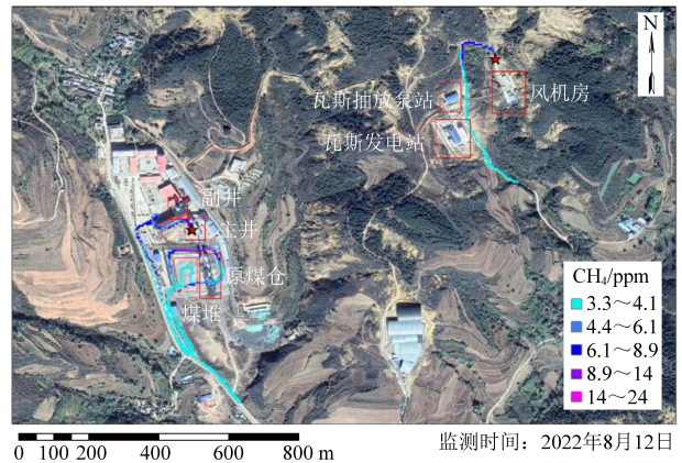
图 2 某煤矿 CH_4 监测浓度空间分布 ( 0.000 1^{\circ} \times 0.000 1^{\circ} , 星号代表下风向静止监测点位置)
