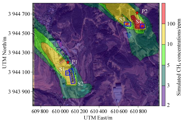
图3 某煤矿CH 4 模拟浓度分布(S1-S3代表排放源位置,星号P1和P2代表受体点位)
