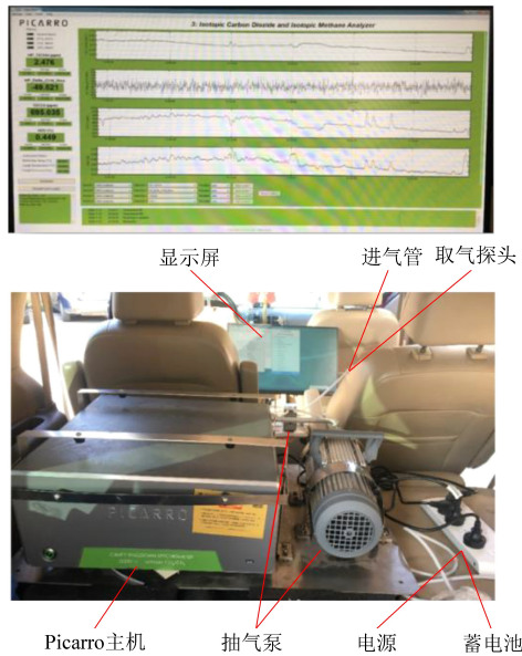
图 1 Picarro 监测设备组成
