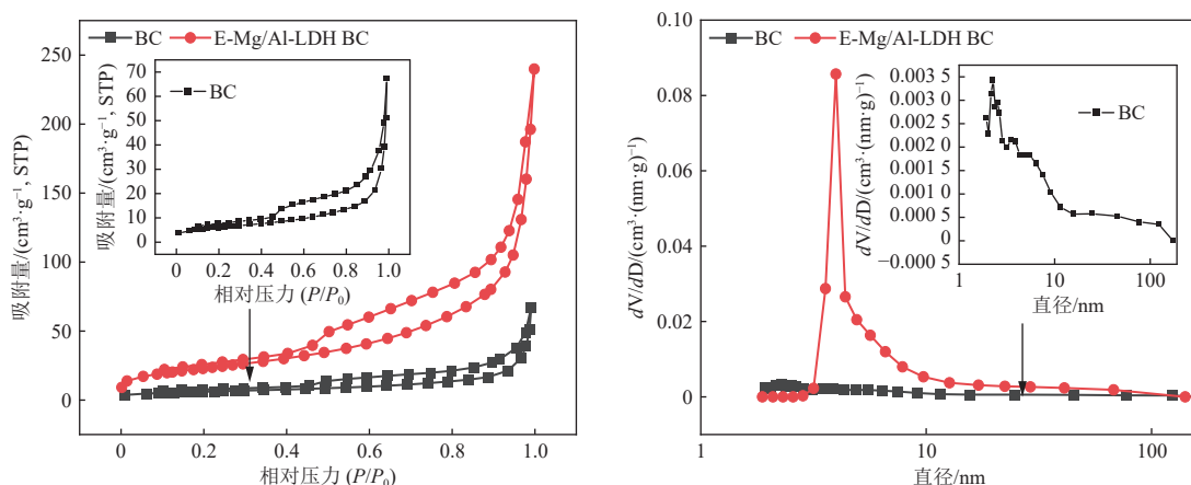
图2 N 2 吸附/解吸等温线和孔径分布
