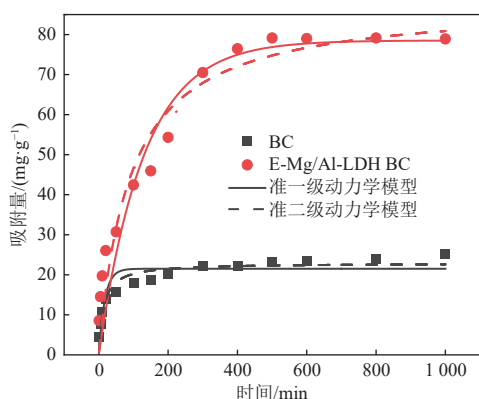
图5 BC、E-Mg/Al-LDH BC 吸附 Ni(II) 的反应动力学特征
