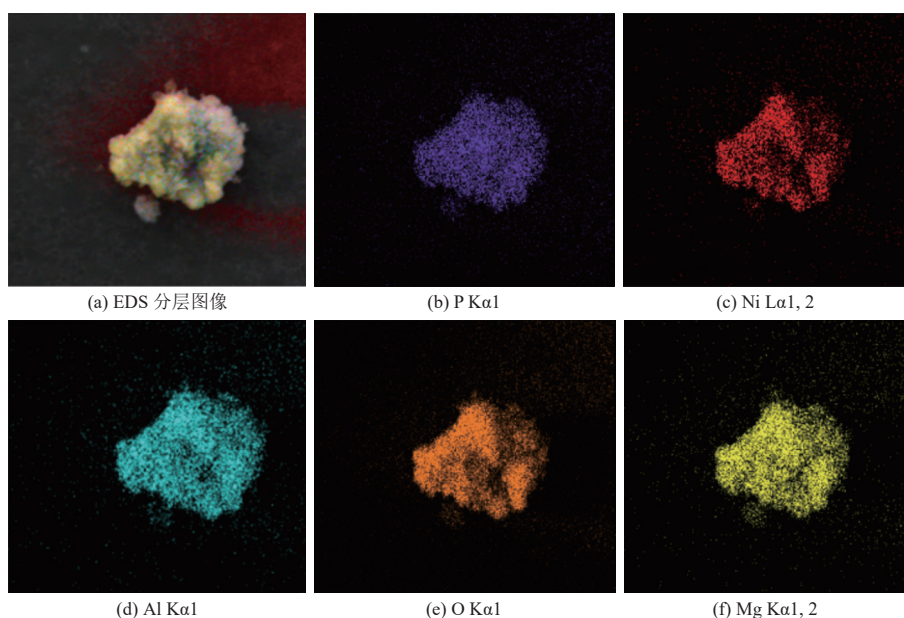
图 8 E-Mg/Al-LDH BC 吸附 Ni(II) 后的 SEM-EDS
