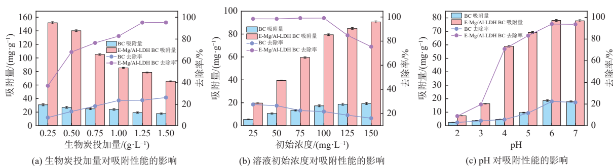
图4 吸附条件对生物炭吸附 Ni(II) 性能的影响
