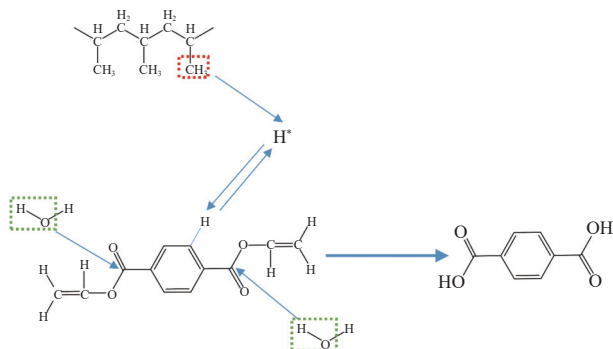
图 4 蒸汽辅助共热解 PET 和 PP 制备 TPA 的反应机理 [62]
