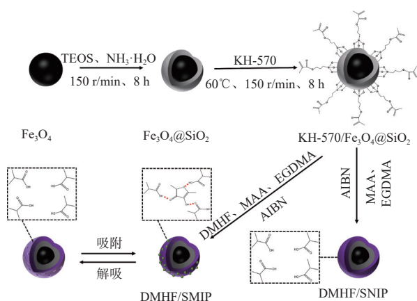
图1 磁性分子印迹聚合物 DMHF/SMIP 的制备流程
