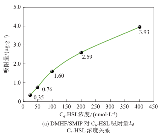
图 6 DMHF/SMIP 对 C_6 -HSL 吸附
