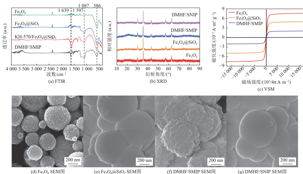
图 2 材料表征
