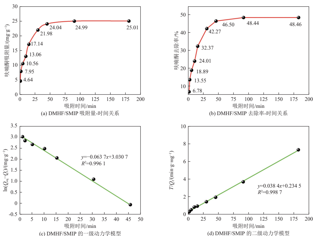
图 3 DMHF/SMIP 吸附动力学及模型拟合
