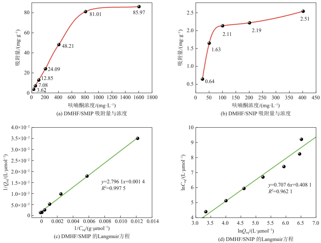
图 4 DMHF/SMIP 吸附热力学及模型拟合
