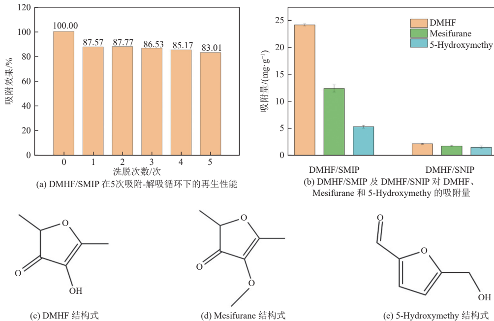
图 5 重复吸附及选择性吸附实验
