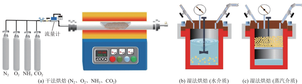
图1 生物质烘焙预处理装置和分类
