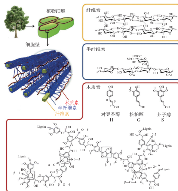
图1 木质纤维素类生物质结构与其三大组分 [7]
