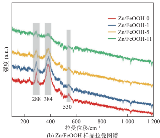
图 2 Zn/FeOOH 样品的 XRD 与拉曼图谱
