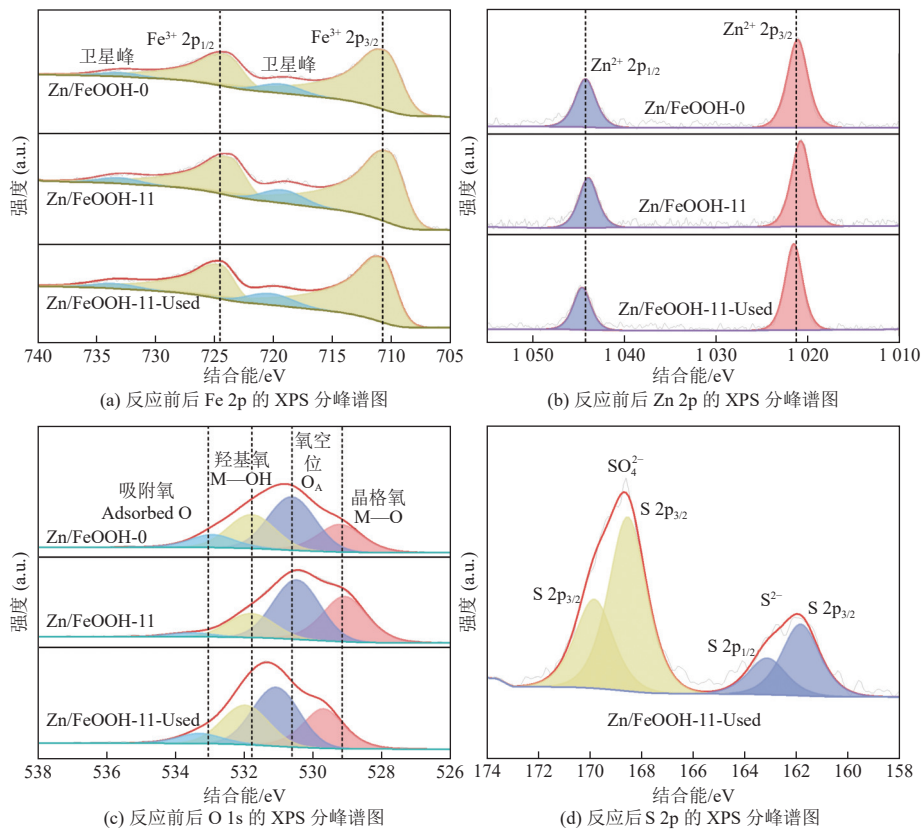
图 5 Zn/FeOOH 样品反应前后 Fe 2p、Zn 2p、O 1s、S 2p 的 XPS 分峰谱图
