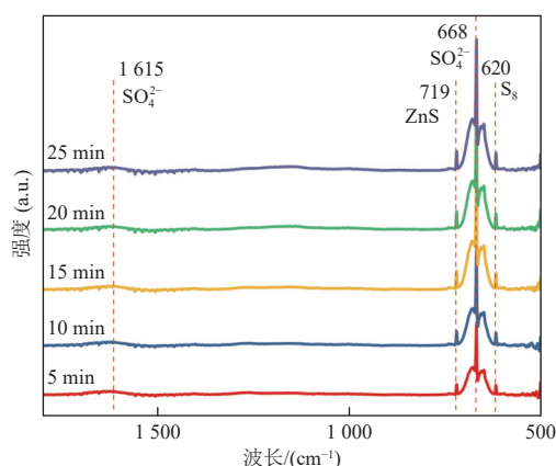
图 6 Zn/FeOOH-11 样品的原位红外光谱图
