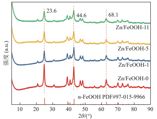
(a) Zn/FeOOH 样品的 XRD 图谱
