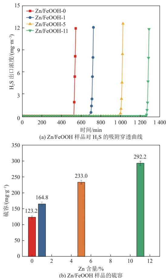
图 1 Zn/FeOOH 样品对 H 2 S 的吸附穿透曲线及硫容
