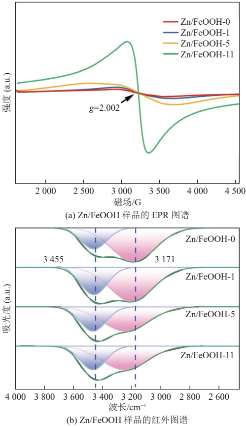
图 4 Zn/FeOOH 样品的 EPR 与红外图谱 Fig. 4 EPR and infrared spectra of Zn/FeOOH
