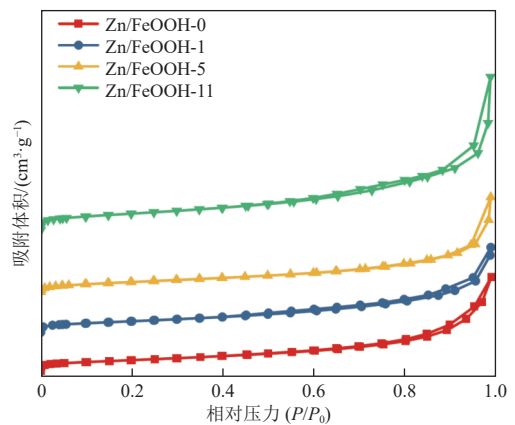
图 3 Zn/FeOOH 样品的 \text{N}_2 吸脱附曲线
