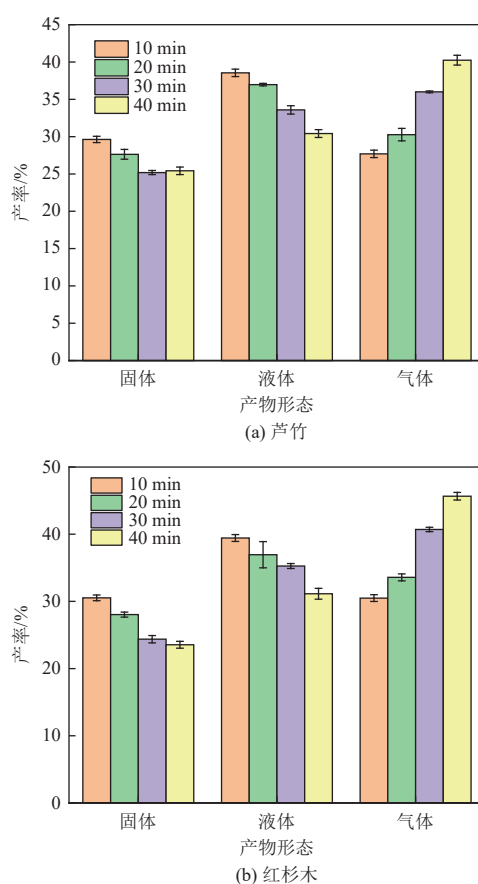
图4 生物质热解三态产率随热解时间的变化
