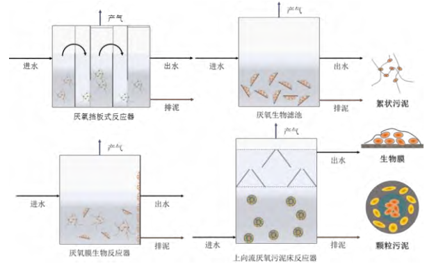
图 2 第二代厌氧消化技术示意图
