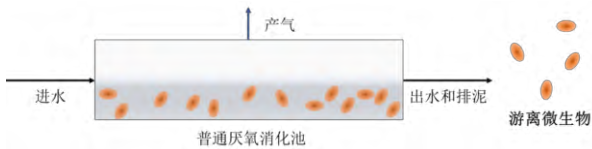
图1 第一代厌氧消化技术示意图
