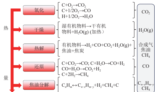
图2 气化过程主要反应 [22-23]
