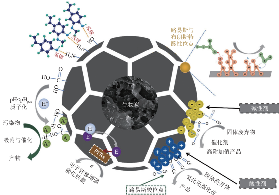
图 6 生物炭催化剂催化转化有机固废机理示意图 [1]
