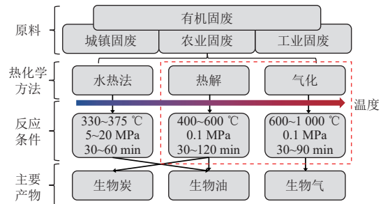
图1 有机固废热化学处理技术 [21]
