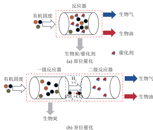
图3 热解气化过程示意图 [38-39]
