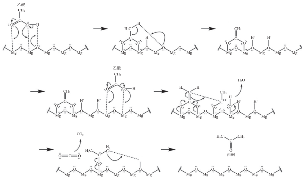
图 4 羧酸的酮基化反应示意图 [43]
