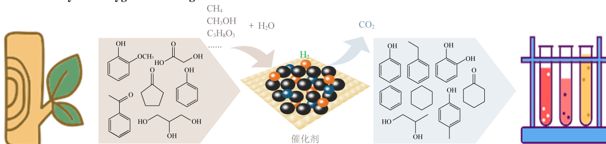
图2 木质素联合水相重整加氢脱氧机理 Fig. 2 RHDO mechanism of lignin
