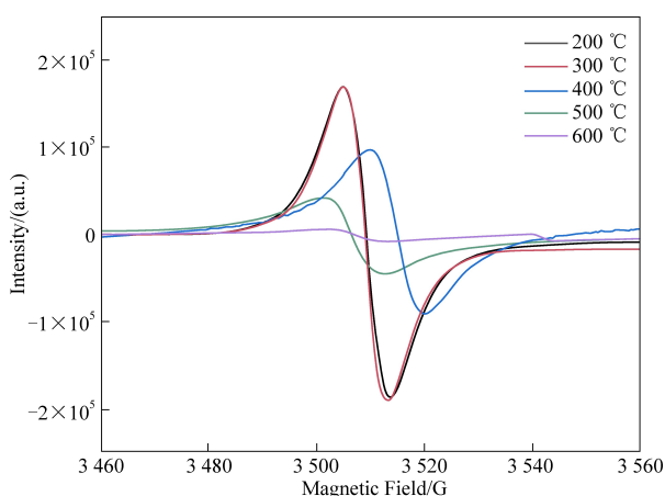
图3 200~600 °C对污泥热化学处理的EPR光谱图
