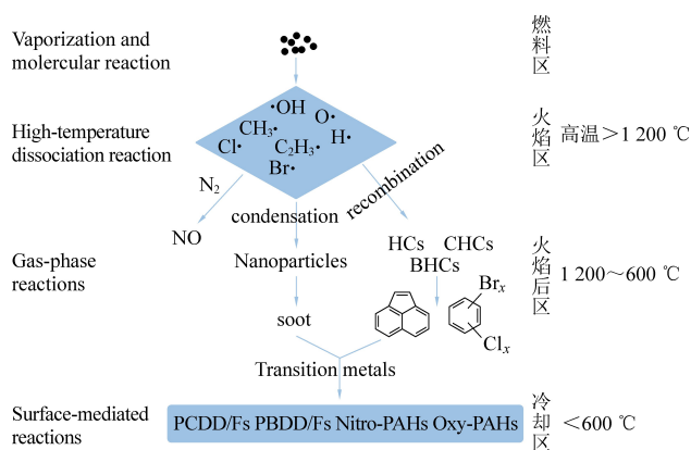
图4 燃烧反应系统不同温度区域的有机热化学反应
